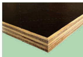
Contreplaqué filmé (15mm 7 plis) PIN MARITIME
